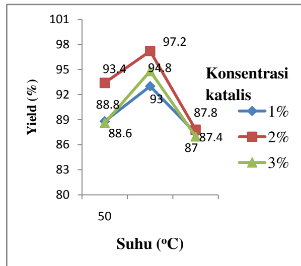
Gambar 3.1 Grafik hubungan antara yield biodiesel terhadap suhu pada variasi konsentrasi katalis
