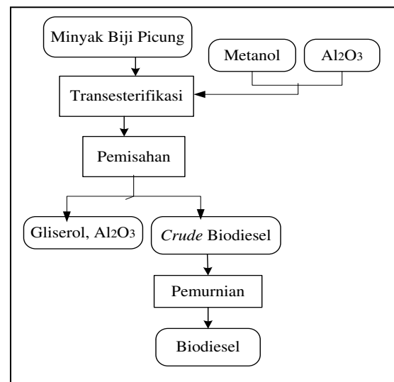
Gambar 2.3 Pembuatan Biodiesel
