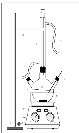
Gambar 2.1 Rangkaian Alat Transesterifikasi
