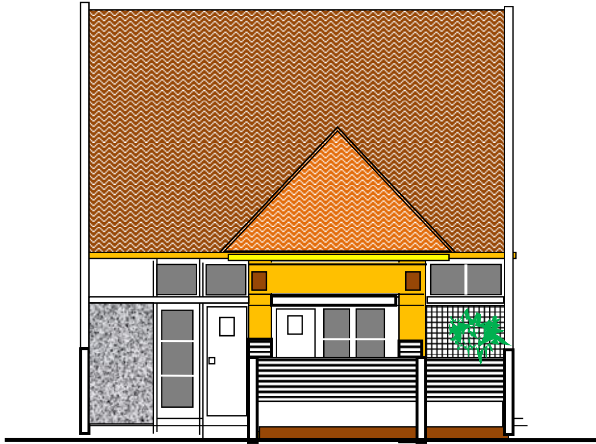
TAMPAK DEPAN 1:100
