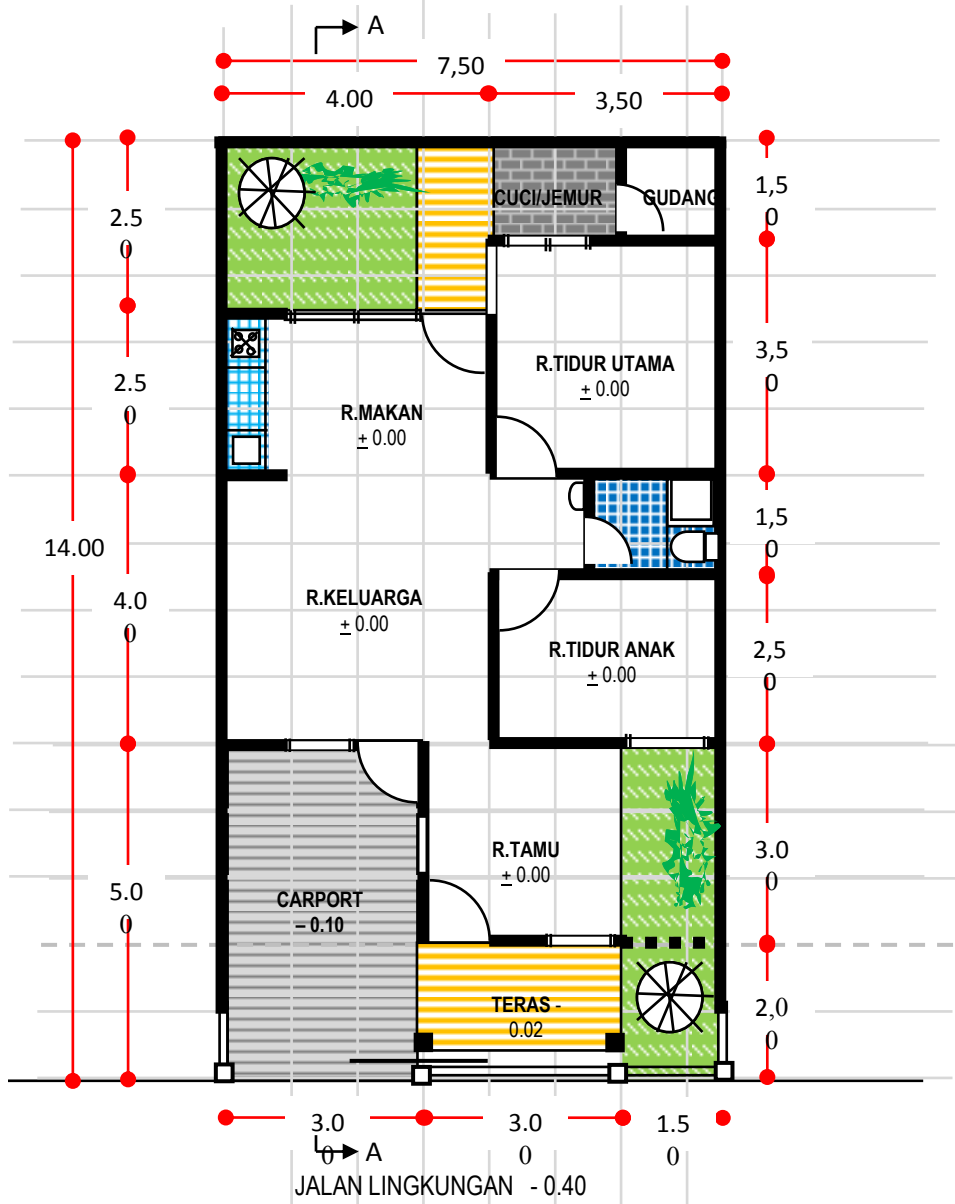
DENAH SITUASI 1:100
